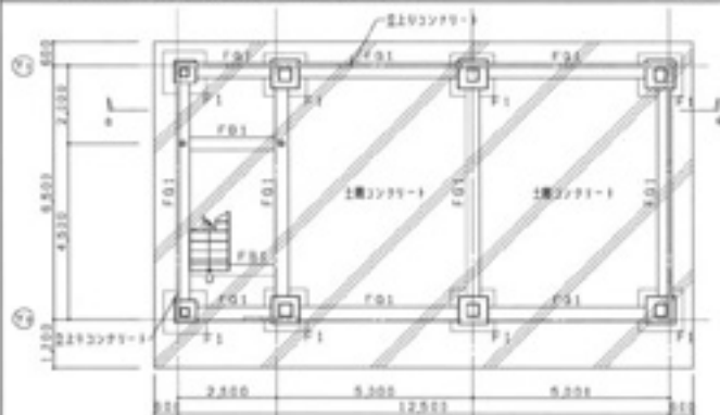
基礎伏図
