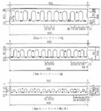
スパンクリートの標準製品の種類と形状
