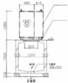
正面図
