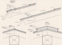
圖 10 屋頂 構造
