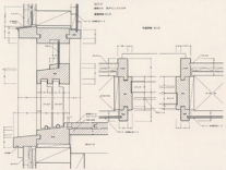
圖例 窗框剖面圖
