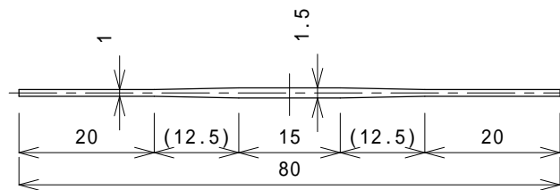
車軸、竹籤 テーパ削り
