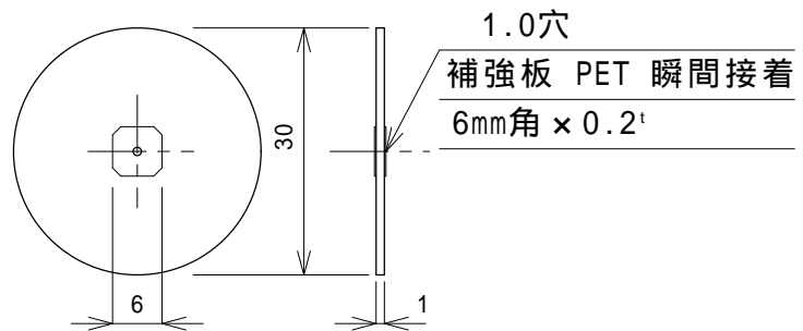
車輪 × 2枚、1mmバルサ ( C カット材 )
